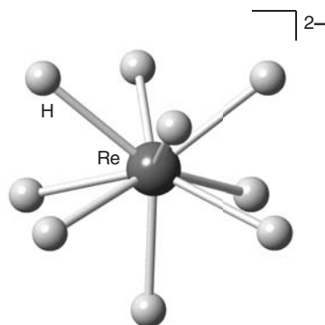
8 [\text{ReH}_9]^{2-}
