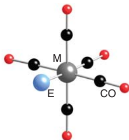
23 [M(CO)_5E] , E = Ar, Kr, Xe
