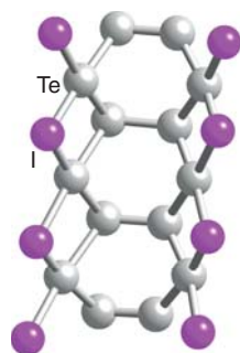
1 \text{Te}_2\text{I}
