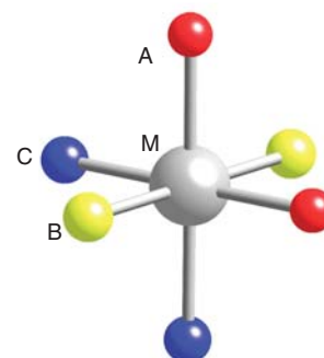
61 [MA 2 B 2 C 2 ]
