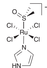
6 NAMI-A
