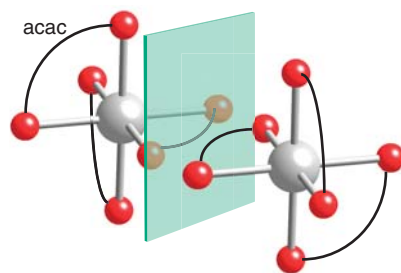
67 [Mn(acac) 3 ] enantiomers
