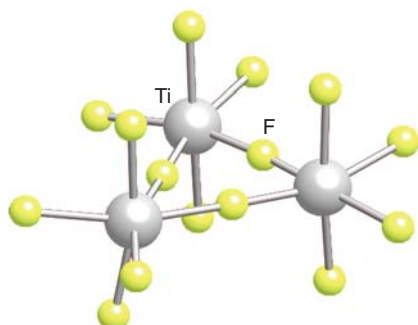
8 \text{Ti}_3\text{F}_{15}
