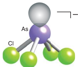
16 \text{AsCl}_4^-
