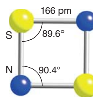
12 \text{S}_2\text{N}_2
