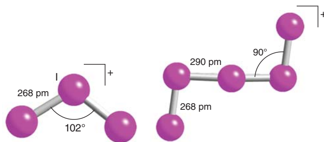
4 I 3 + , C 2v
