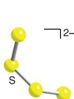
34 \text{S}_2^{2-}
