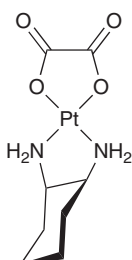
3 Oxaliplatin
