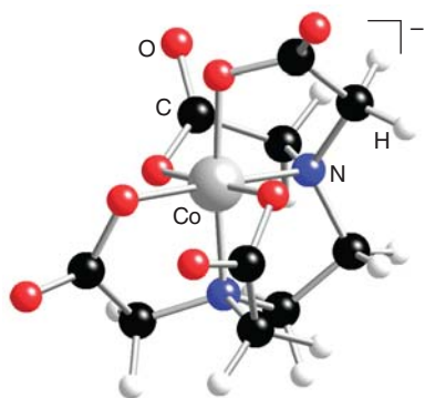
7 [Co(edta)] -
