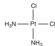
1 Cisplatin
