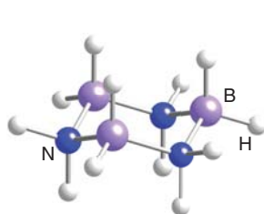
21 \text{N}_3\text{B}_3\text{H}_{12}
