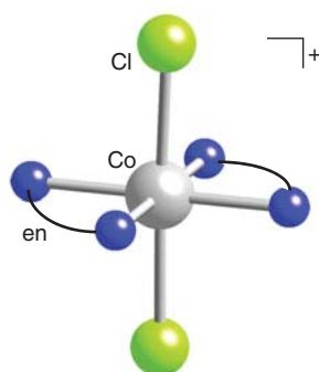
69 trans -[CoCl 2 (en) 2 ] +
