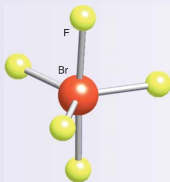
11 BrF 5 , D 3h
