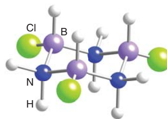
24 \text{B}_3\text{N}_3\text{H}_9\text{Cl}_3
