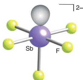
17 \text{SbF}_5^{2-}
