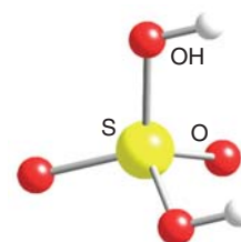
5 O_2S(OH)_2 , H_2SO_4
