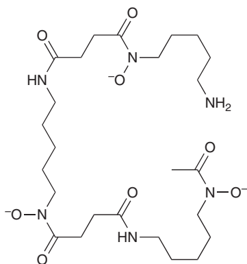
25 Desferral
