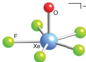
14 \text{XeOF}_5^-
