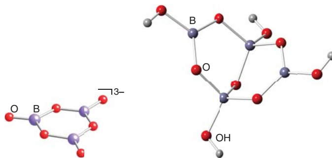
18 [B_3O_6]^{3-}
