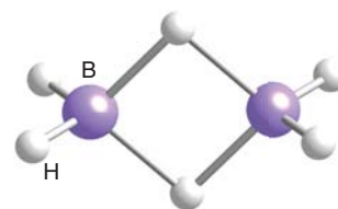
4 Diborane, \text{B}_2\text{H}_6
