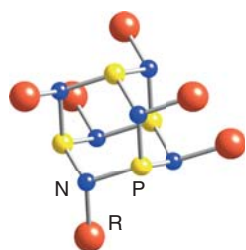
25 \text{P}_4(\text{NR})_6
