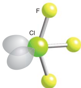
1 ClF 3 , C 2v
