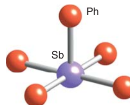
38 Sb(C_6H_5)_5
