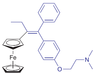
11 Ferrocifen
