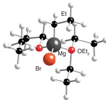
12 MgEtBr(OEt 2 ) 2
