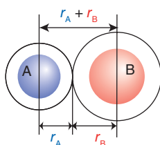
20 van der Waals radius
