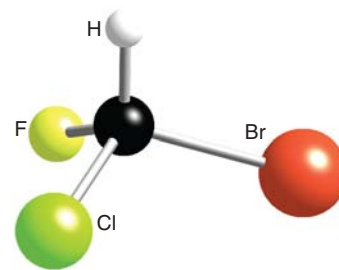
12 \text{CHClFBr} , C_1
