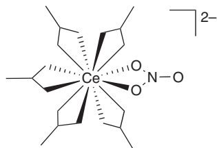
33 [\text{Ce}(\text{NO}_3)_6]^{2-}
