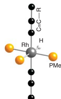
65 mer-trans -[RhH(C≡CR) 2 (PMe 3 ) 3 ]
