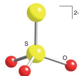
8 \text{S}_2\text{O}_3^{2-}
