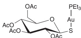
17 Auranofin
