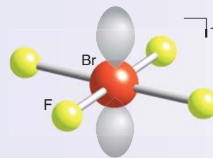
12 BrF 4 −
