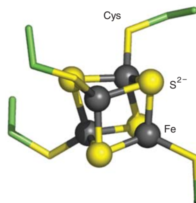
26* [4Fe-4S]
