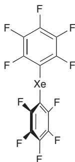
20 Xe(C 6 H 5 ) 2
