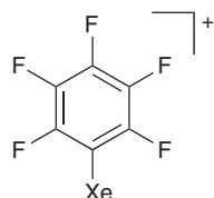
19 C 6 F 5 Xe +
