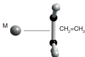
32 \eta^2\text{-CH}_2=\text{CH}_2
