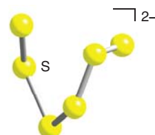
35 \text{S}_6^{2-}
