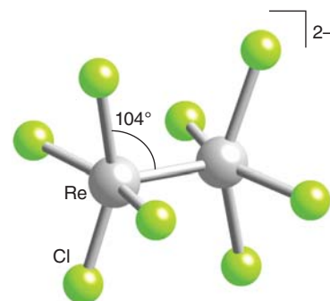
11 [\text{Re}_2\text{Cl}_8]^{2-}
