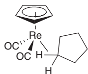
65
