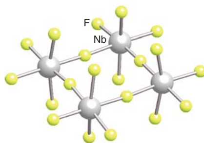
9 \text{Nb}_4\text{F}_{20}
