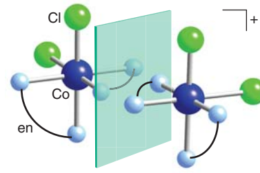
68 cis -[CoCl 2 (en) 2 ] + enantiomers
