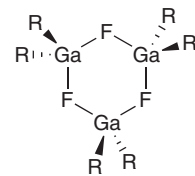
42
