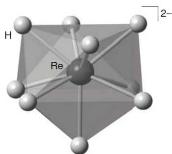
32 [\text{ReH}_9]^{2-}
