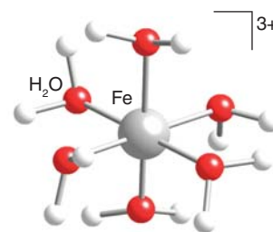
3 [Fe(OH_2)_6]^{3+}
