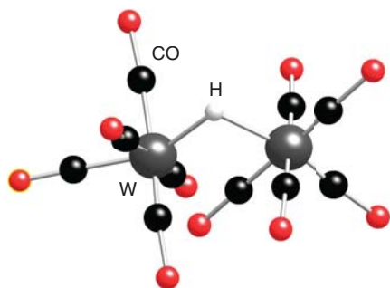
7 [(\text{CO})_5\text{W}-\mu\text{H}-\text{W}(\text{CO})_5]^{2-}
