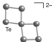
36 \text{Te}_8^{2-}
