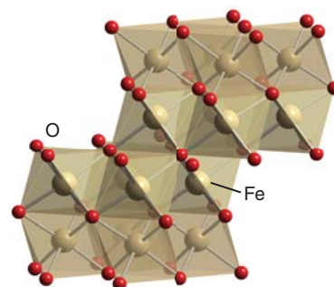
20 Ferrihydrite
