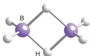
1 Diborane, B_2H_6
