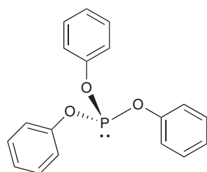
21 P(OPh)_3
