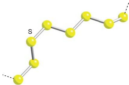
15 S_n
