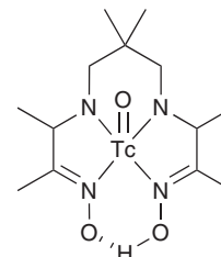
34 Ceretec (brain)
