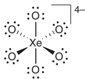
13 \text{XeO}_6^{4-}
