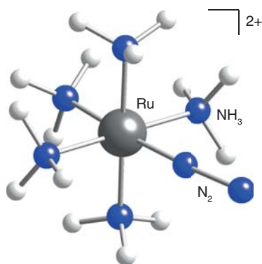
9 [Ru(NH_3)_5(N_2)]^{2+}
