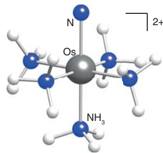
11 [Os(NH_3)_5N]^{2+}
