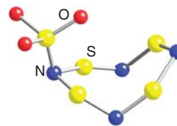
39 S_4N_4SO_3
