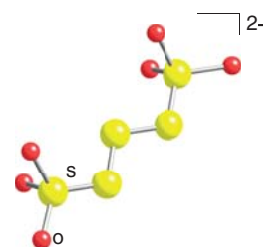
6 Pentathionate ion, \text{S}_5\text{O}_6^{2-}
