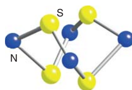
11 \text{S}_4\text{N}_4
