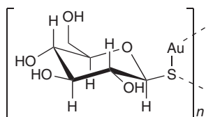
16 Solganol
