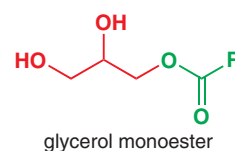
glycerol monoester
