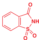
saccharin
