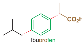
ibuprofen
