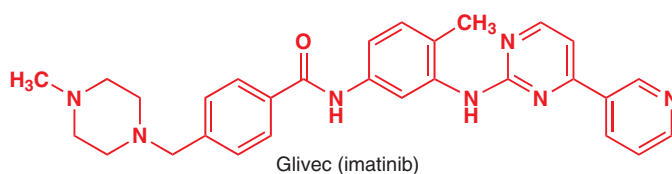
Glivec (imatinib)
